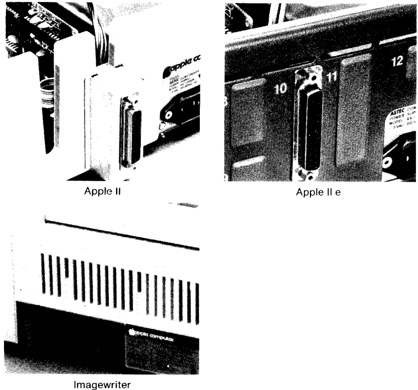
Figure 1-2. Connecteurs d'interface série de l'Apple II/IIe
