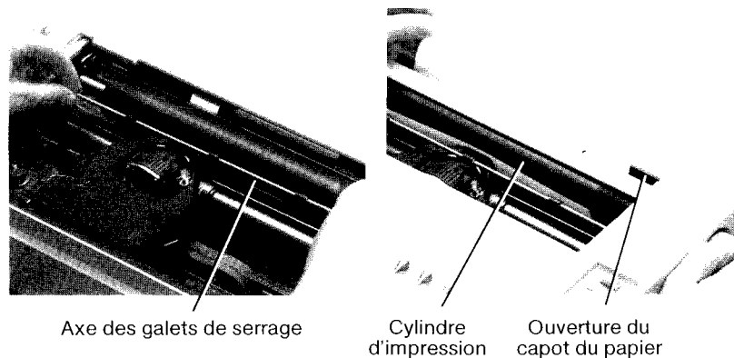
Figure 2-6. Chargement de papier ordinaire
