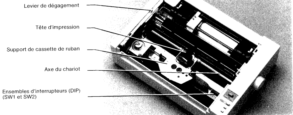
Figure 1-7. Pièces internes
