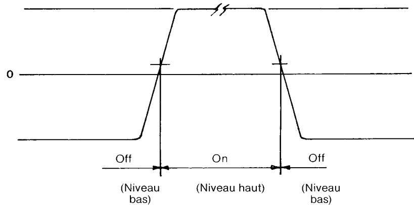
Figure F-4. Niveau de tension de seuil
