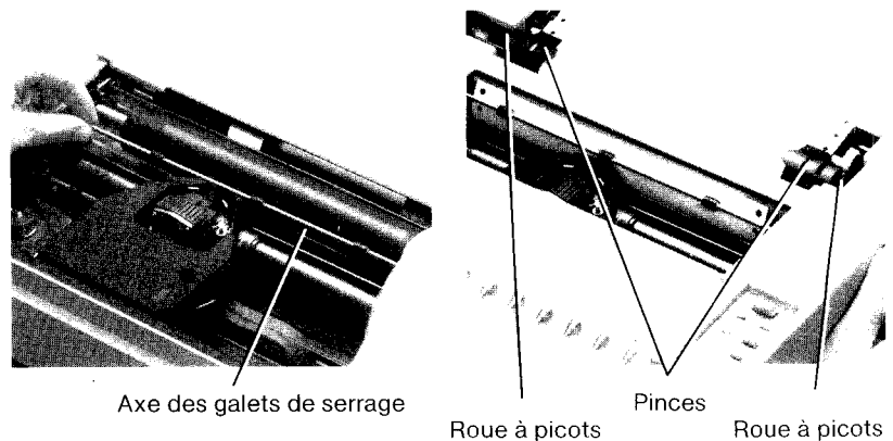
Figure 2-4. Chargement du papier entraîné par picots
