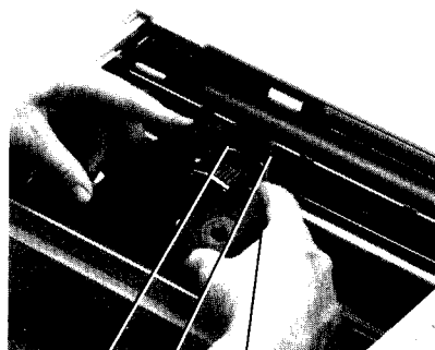
Support de la cassette Plaque métallique Guide du ruban
