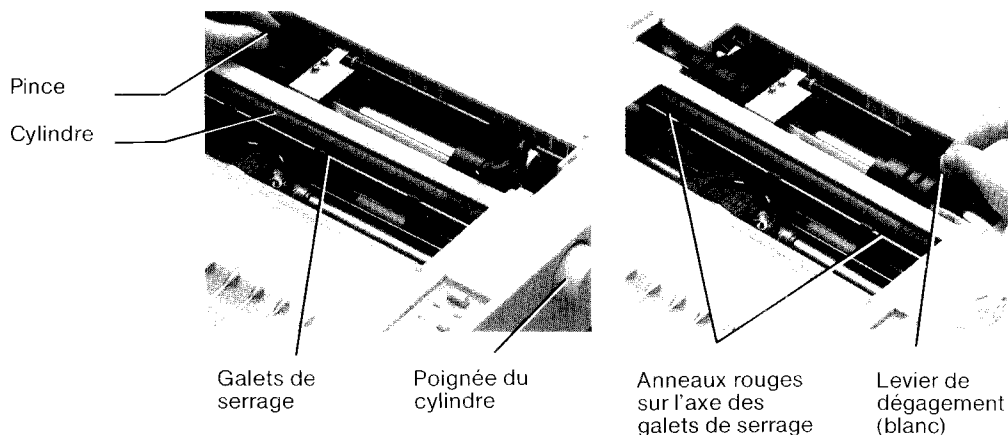
Figure 2-3. Réglage des roues à picots
